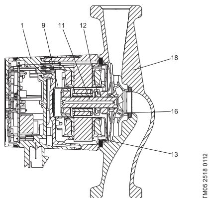
Рис. 14. Насос ALPHA2/ALPHA2 L
