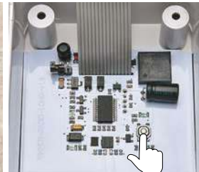
Фото 15. Нажмите кнопку SET/RESET электропривода
