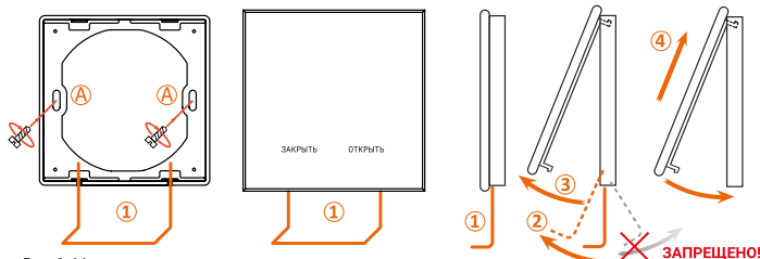
Рис. 1. Монтаж, установка и снятие сенсорного радиопульта
