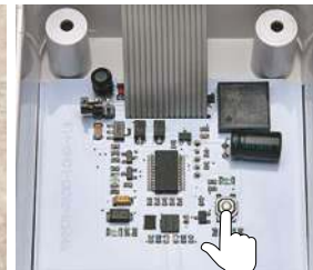
Фото 15. Нажмите кнопку SET/RESET электропривода
