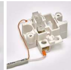
Фото 17. Подключение проводного выключателя
