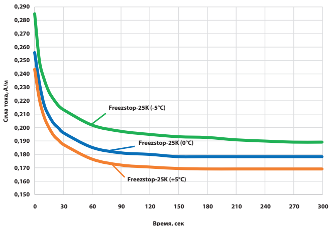
Рисунок 2.4. График зависимости пускового тока (А/м) от времени (сек.) для кабелей Freestop-25K при испытании в воде (+5°C), в талой воде (0°C), во льду (-5°C)
