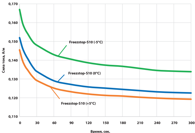
Рисунок 2.2. График зависимости пускового тока (А/м) от времени (сек.) для кабеля Freezstop-S10 при испытаниях в воде (+5°C), в талой воде (0°C), во льду (-5°C)
