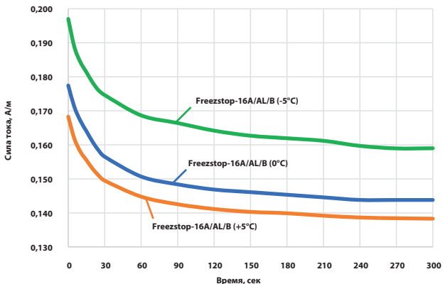
Рисунок 2.3. График зависимости пускового тока (А/м) от времени (сек.) для кабелей Freestop-16A/AL/B при испытании в воде (+5°C), в талой воде (0°C), во льду (-5°C)
