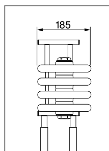
5-трубчатая секция
