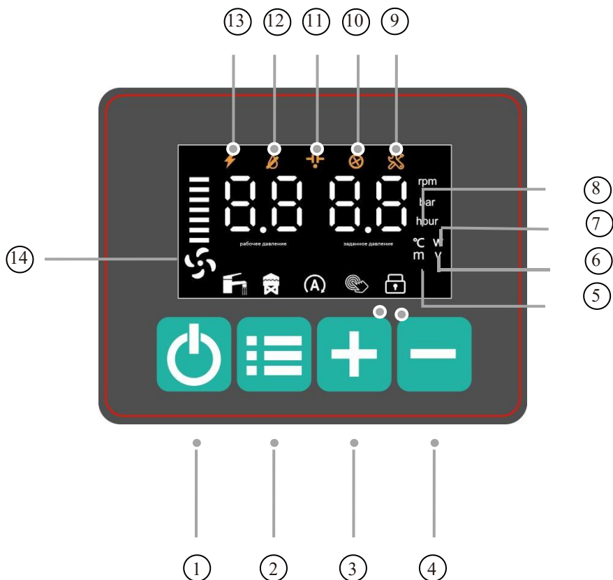
Рис.4. Индикация насосной станции S-BOX4-30
