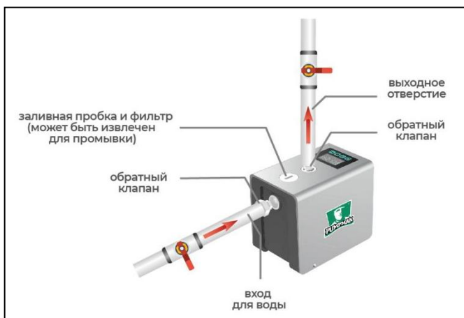
Рис.3. Назначения элементов насосной станции S-BOX4-30
