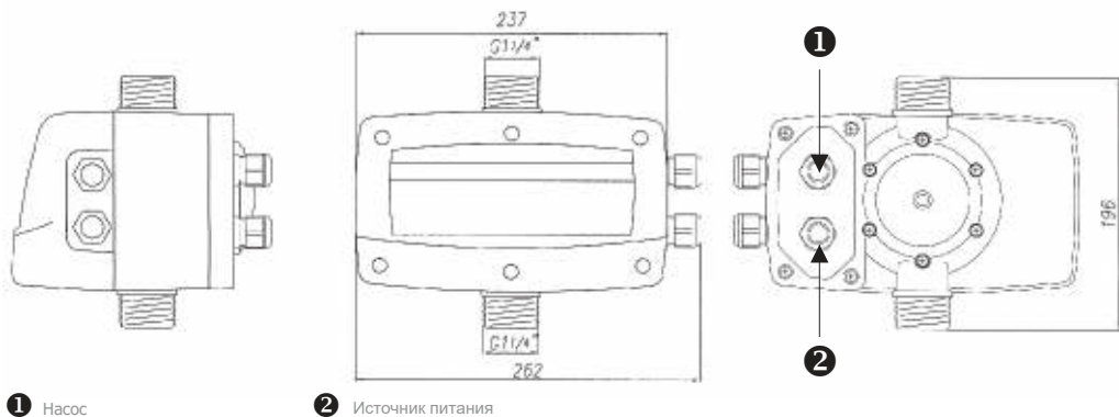
Рис. 2 боковые подключения
